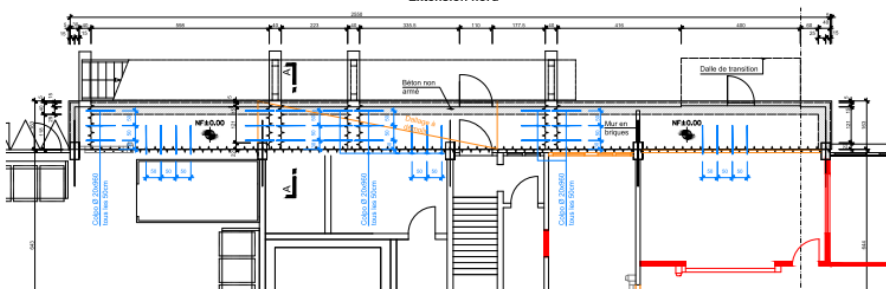
Vue en plan radier 1 1:50 Extension nord
