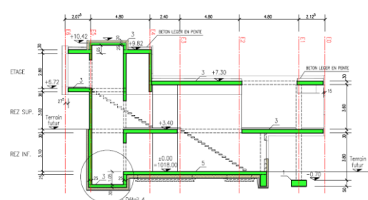
COUPE B-B 1:100
